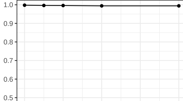
GSE25097
