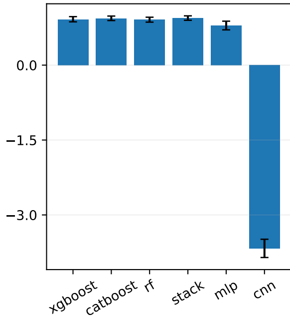
R^2
