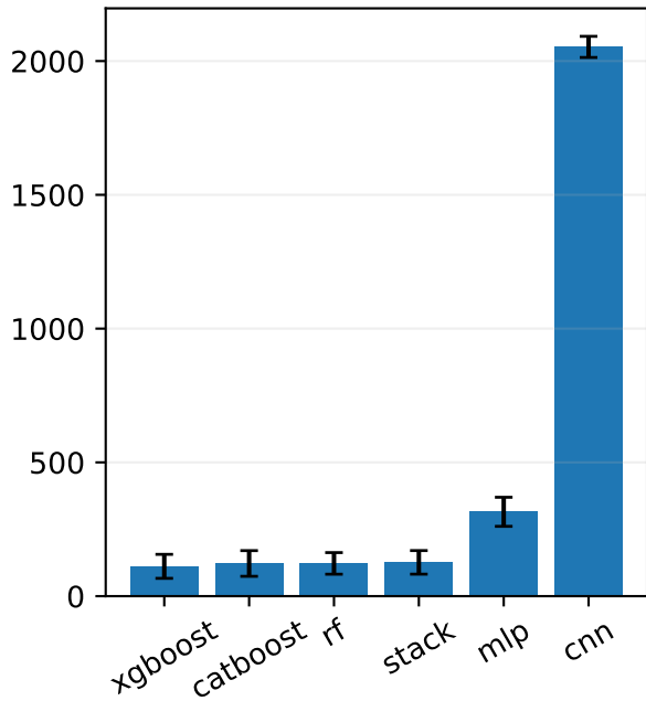
MAE
