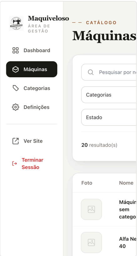
Figura 2 — Lista de máquinas do backoffice a 375 px: a barra lateral ocupa 288 px e a tabela fica cortada (scrollWidth 1156 px).
