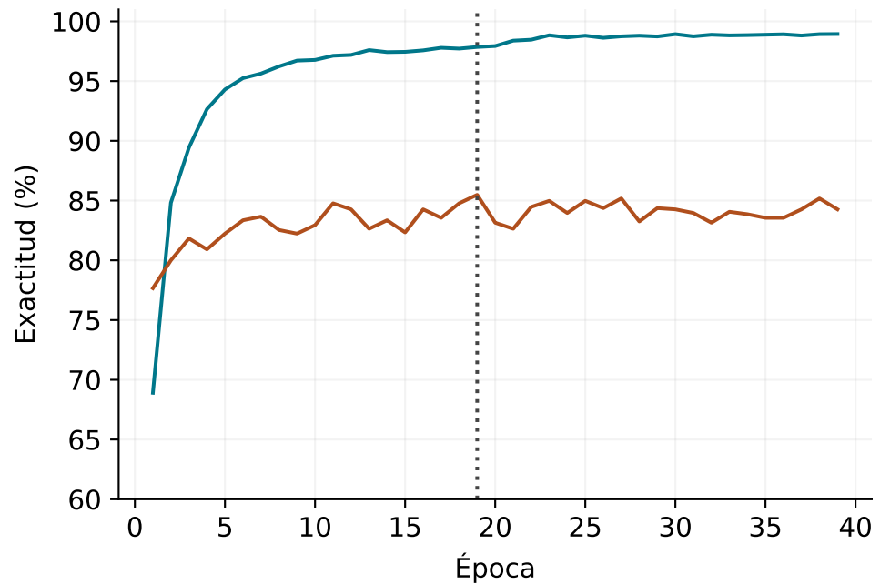
(b) Resolución 64^3
