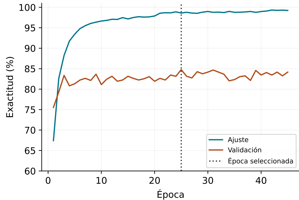
(a) Resolución 32^3
