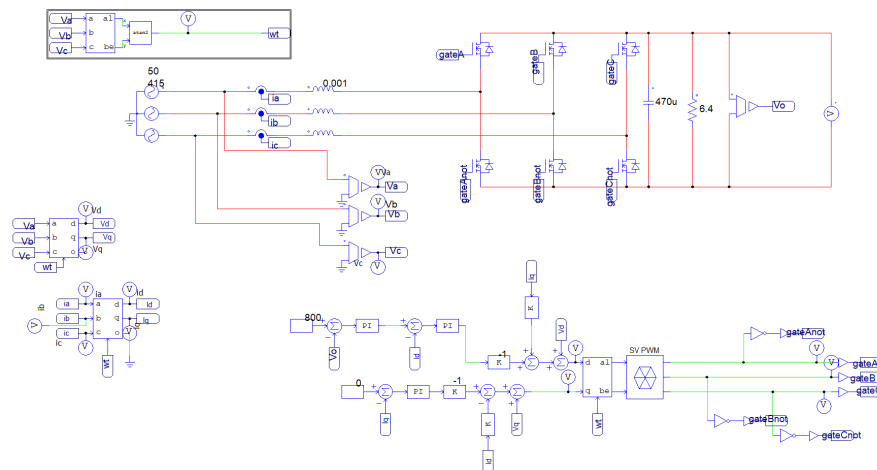
Figura 10 – Diagrama de simulação do retificador PFC trifásico no PSIM.
