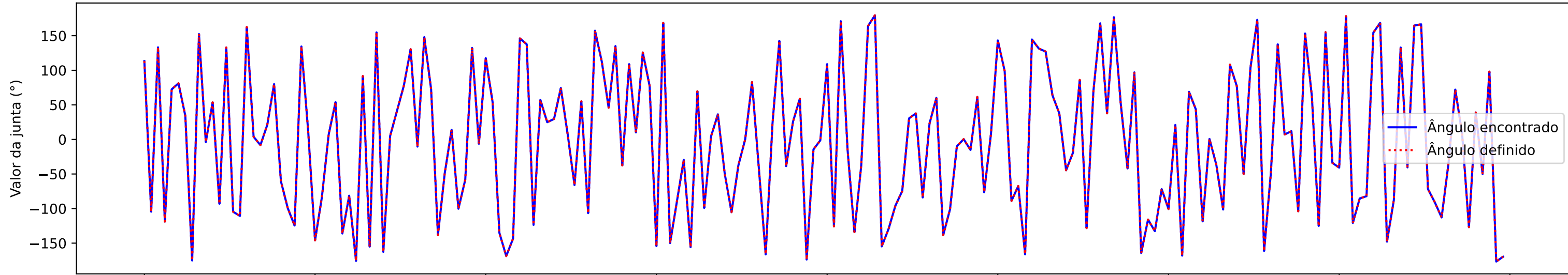
Histórico das variáveis das juntas - q2
