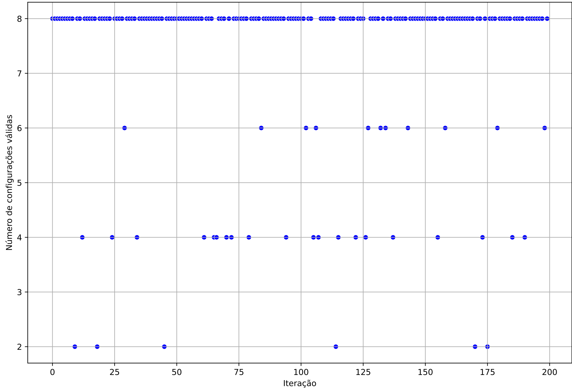
Número de configurações válidas encontradas para o UR5 vs Iteração.
