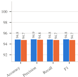
AG News
