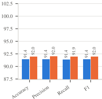
SST 2
