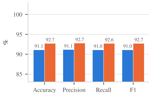
SST 2
