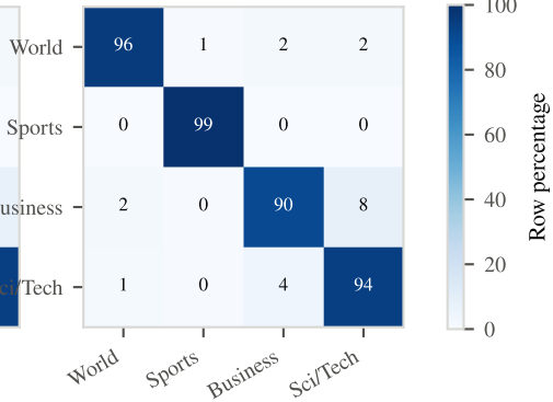
BERT
