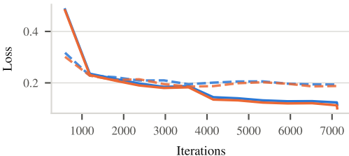
AG News
