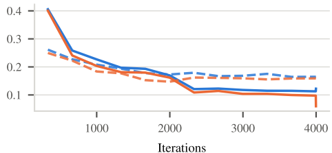
SST 2
