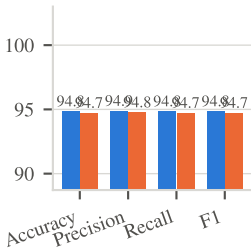
AG News
