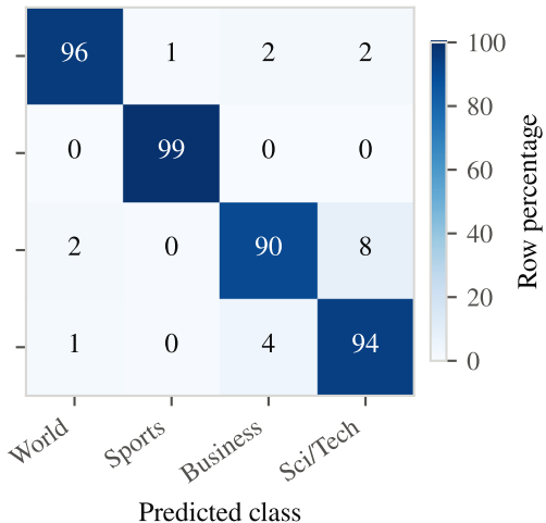
BERT
