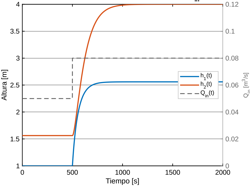
Experimento 2: Respuesta dinamica ante un escalon de Q_{in} en t = 500 s
