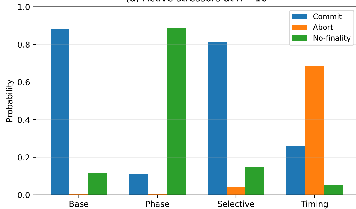
(d) Active stressors at n = 10
