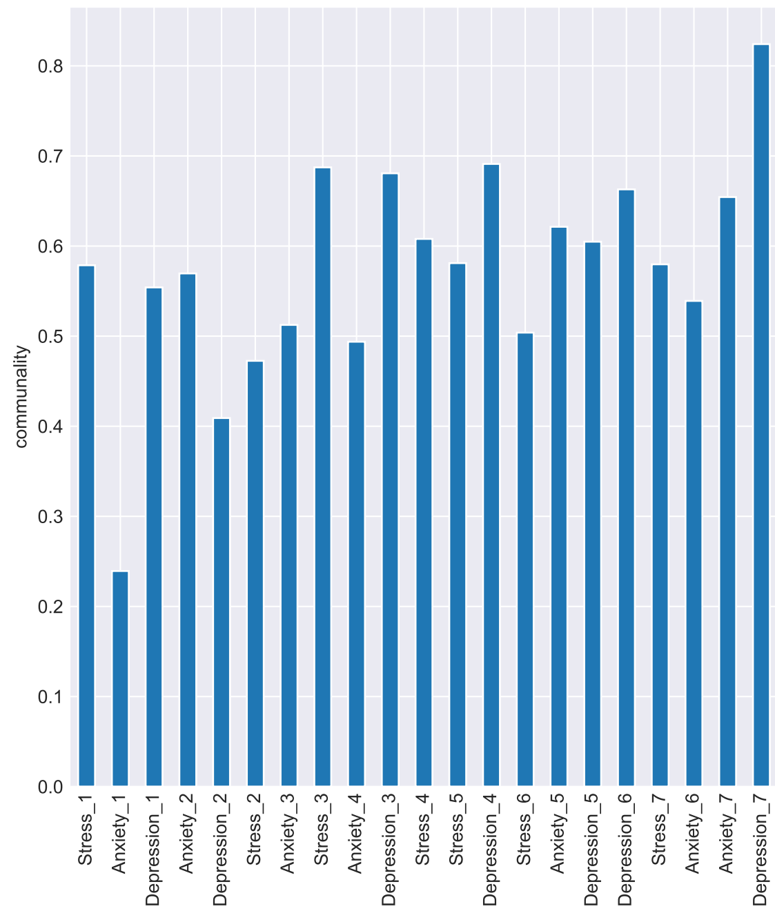
Varimax Rotation
