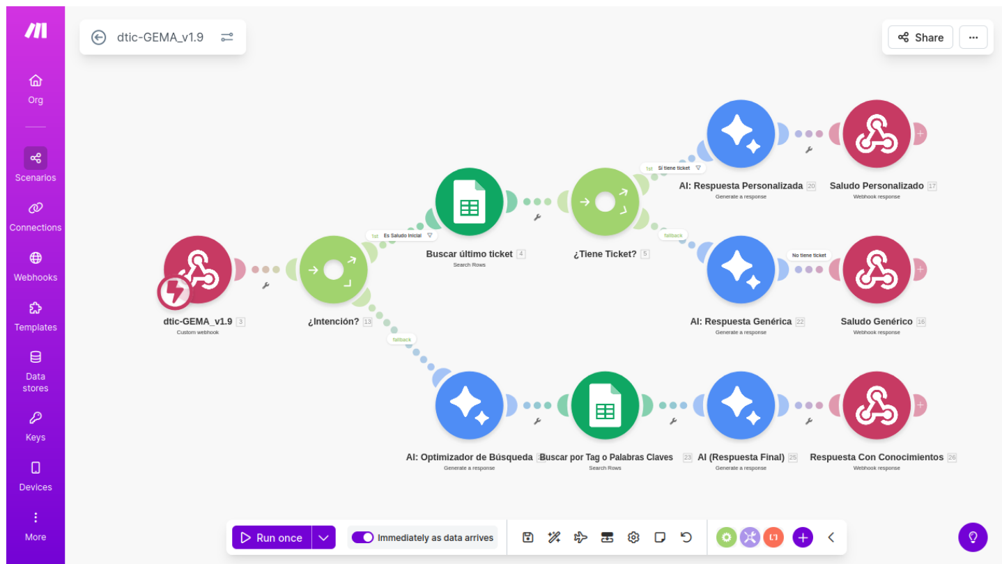
Figura 1: Figura 1: Arquitectura Oficial dtic-GEMA (3 Capas).
