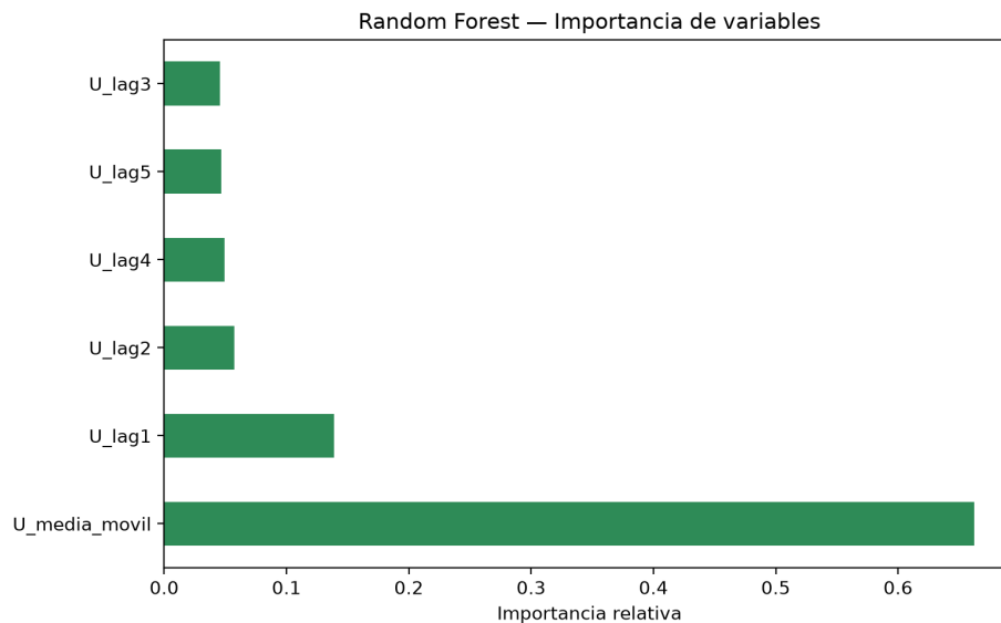
Figura 5.13: Importancia relativa de variables (Impureza de Gini), Random Forest .
