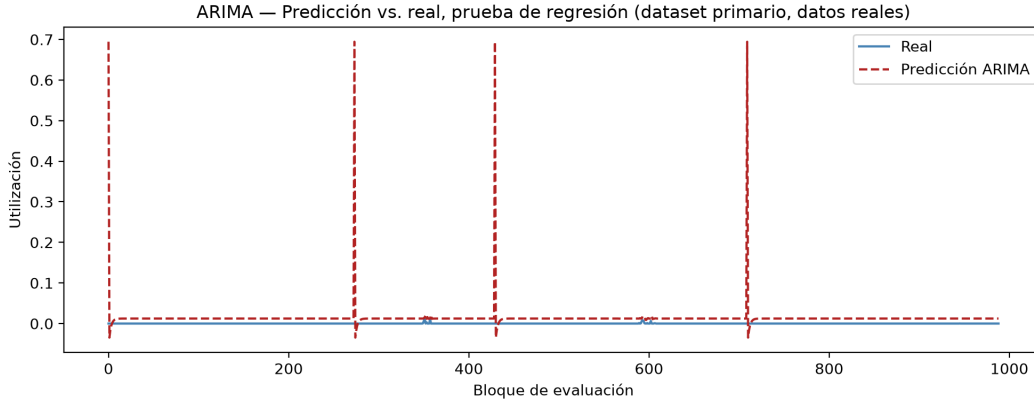
Figura 6.1: ARIMA(3,0,3): predicción vs. valor real, prueba de regresión (dataset primario, datos reales).
