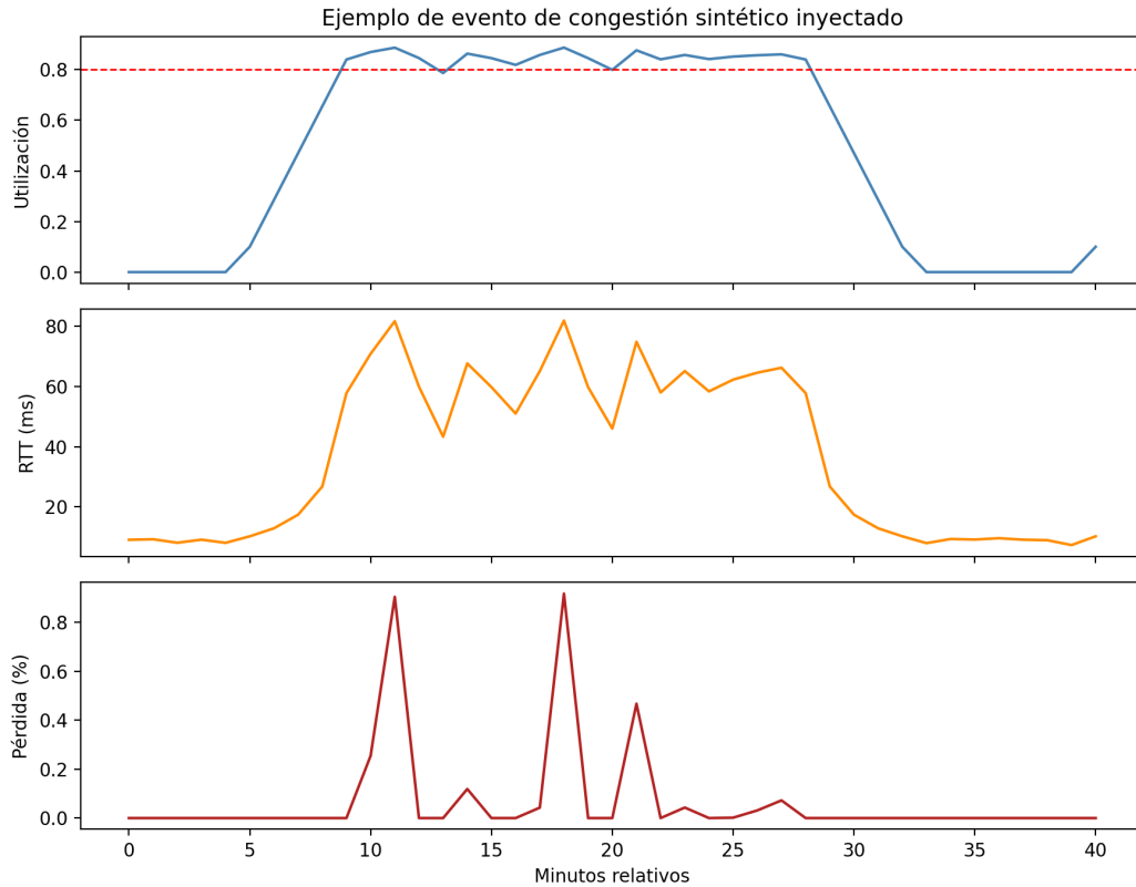
Figura 5.5: Ejemplo de un evento de congestión sintético: utilización, RTT y pérdida de paquetes, derivados mediante el modelo de teoría de colas de la Sección 2.1.3.
