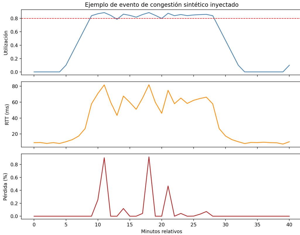
Figura 5.5: Ejemplo de un evento de congestión sintético: utilización, RTT y pérdida de paquetes, derivados mediante el modelo de teoría de colas de la Sección 2.1.2.
