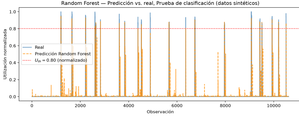
Figura 6.10: Random Forest: predicción vs. valor real, prueba de clasificación (dataset primario, datos sintéticos aislados).
