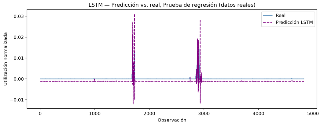
Figura 6.14: LSTM: predicción vs. valor real, prueba de regresión (dataset primario, datos reales).
