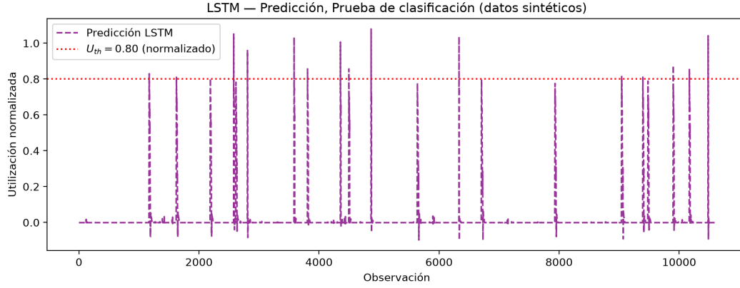
Figura 6.16: LSTM: predicción, prueba de clasificación (dataset primario, datos sintéticos aislados).
