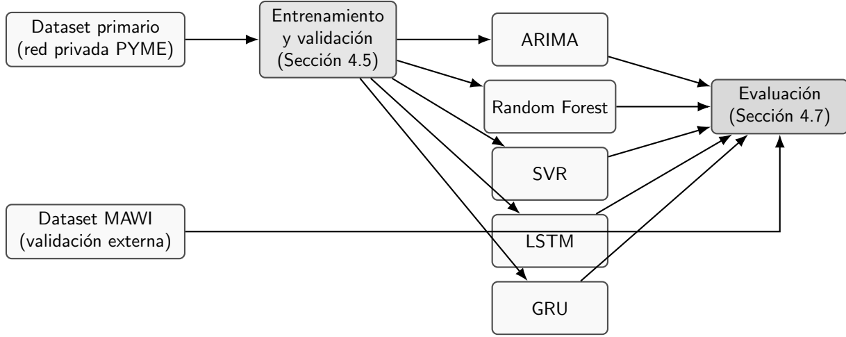
Figura 4.4: Diseño experimental general: entrenamiento sobre el dataset primario y validación cruzada de fuentes contra MAWI.
