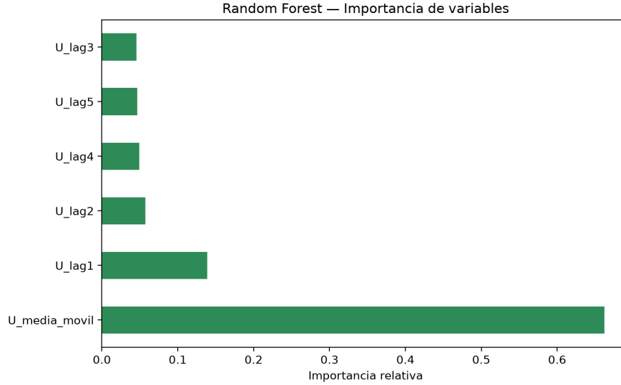
Figura 5.4: Importancia relativa de variables (Impureza de Gini), Random Forest.
