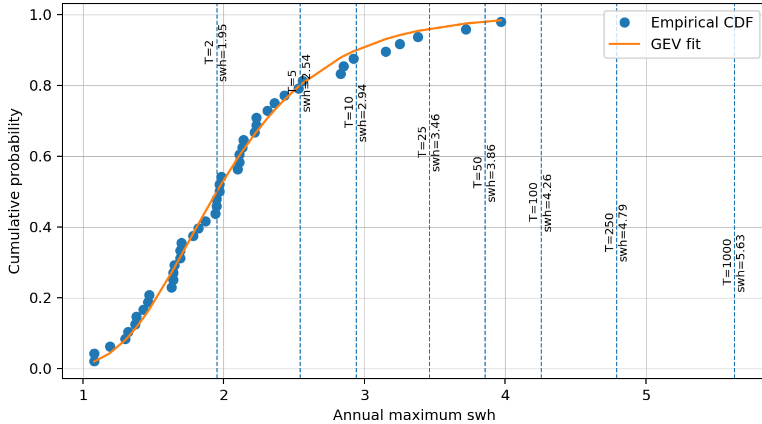
GEV fit: SWH - 090-120
