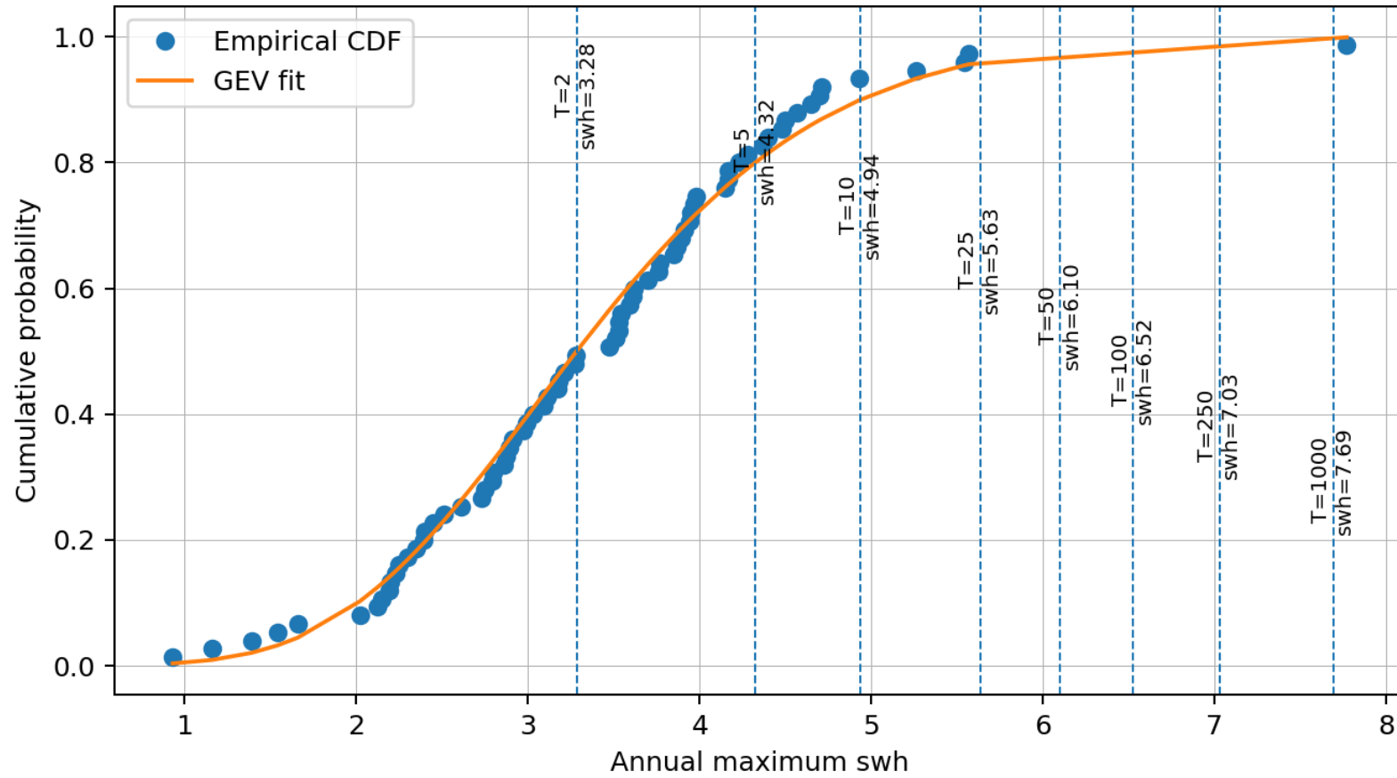
GEV fit: SWH - 150-180
