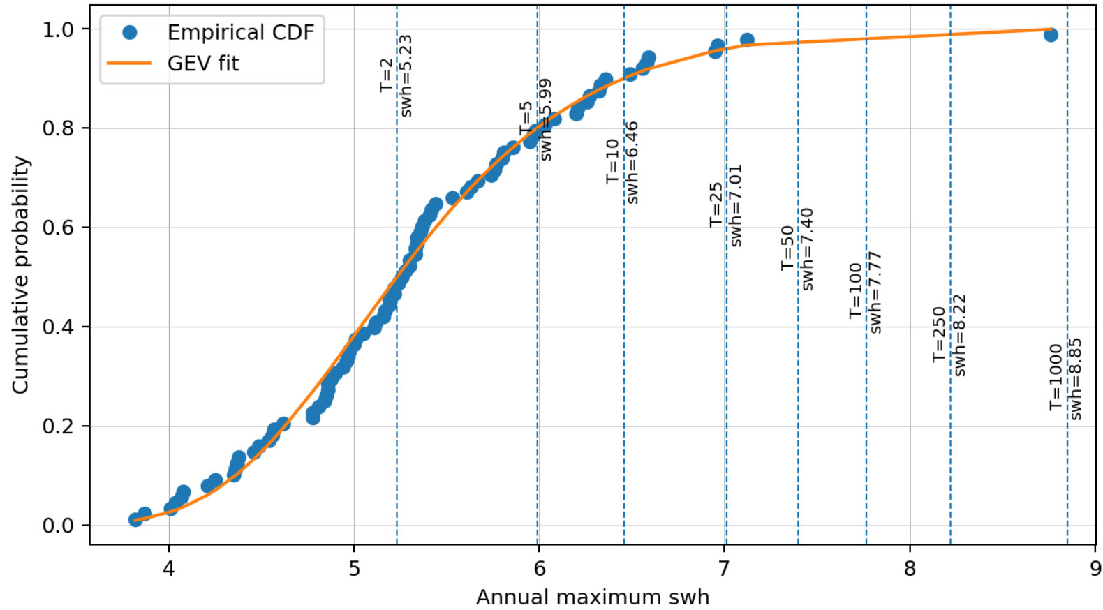
GEV fit: SWH - 330-360
