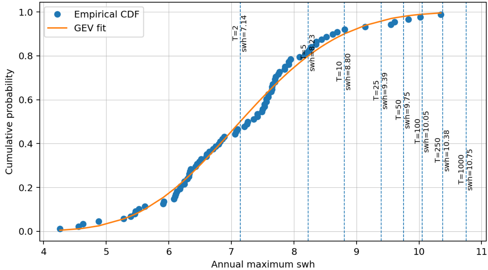
GEV fit: SWH - 270-300
