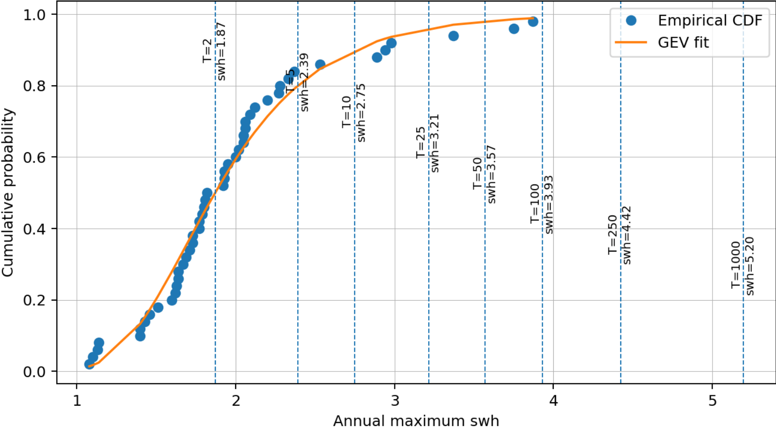
GEV fit: SWH - 060-090
