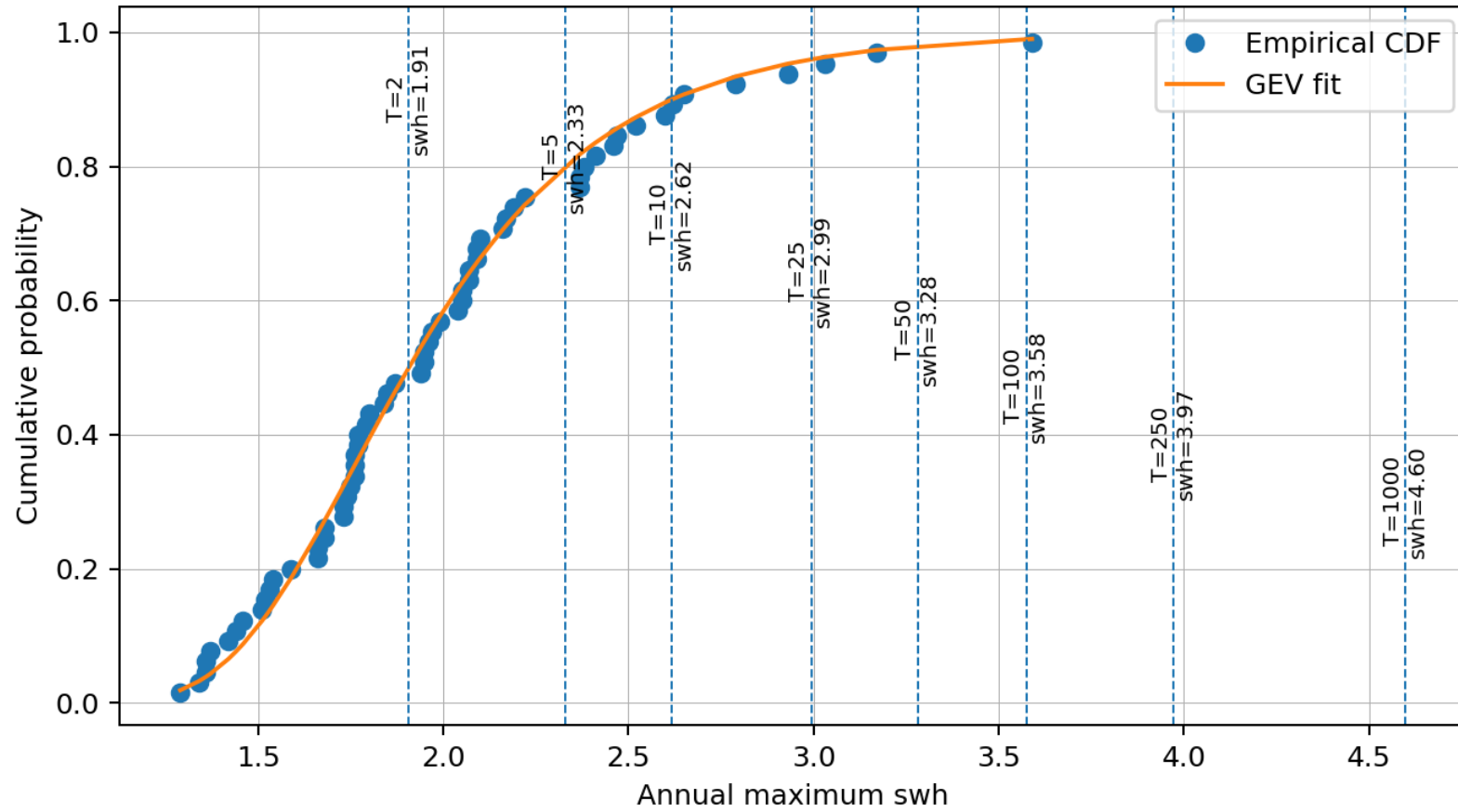
GEV fit: SWH - 030-060
