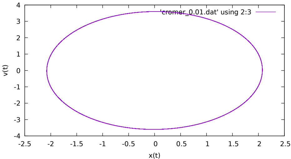
Spazio delle fasi con Eulero-Cromer (dt=0.01)
