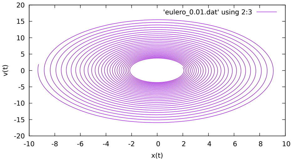
Spazio delle fasi con Eulero (dt=0.01)
