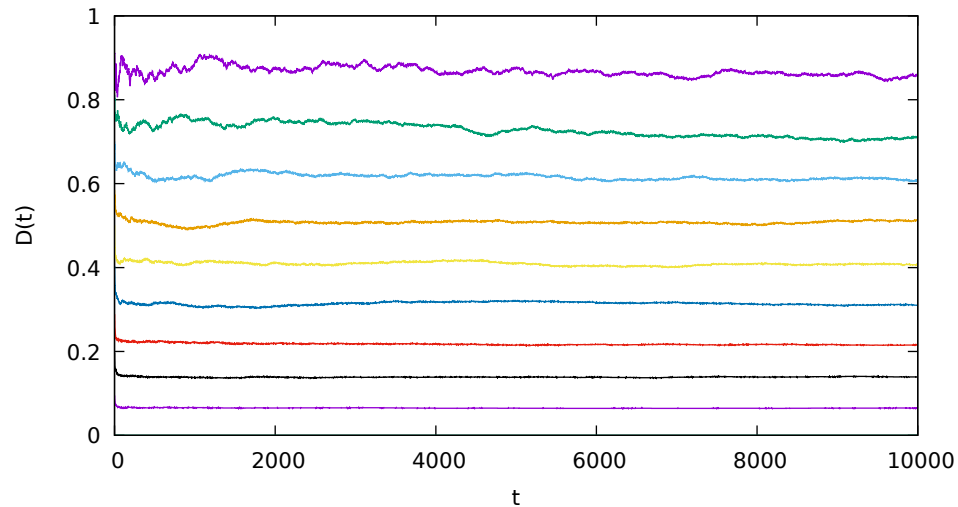
Coeff. di Diffusione per vari Rho (dall alto, 0.1, 0.2, ..., 0.9) [L=100]
