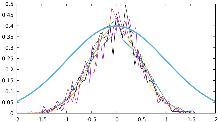
Scaling con istogrammi normalizzati (Traiettorie=1000, Tmax=1000, Base=2)
