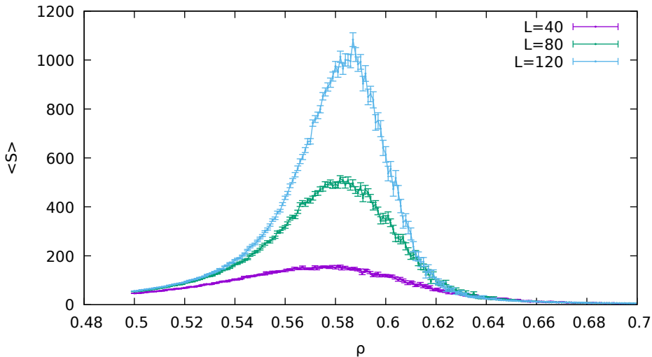
Taglia media dei cluster (Primo Algoritmo, Num Configurazioni=1000)
