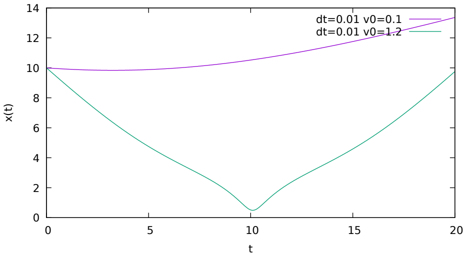
Integratore (algoritmo utilizzato: leapfrog)
