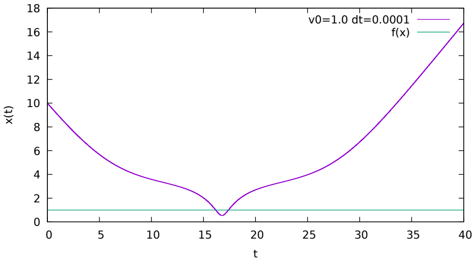
Integratore, vista sugli istanti in cui la particella arriva in x=1 (leapfrog)
