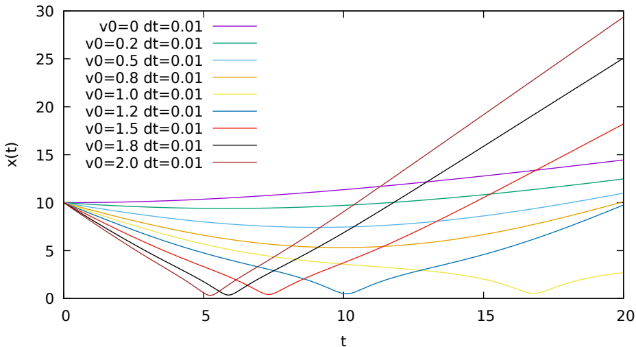
Integratore con varie velocita tra 0 e 20 (algoritmo utilizzato:leapfrog)
