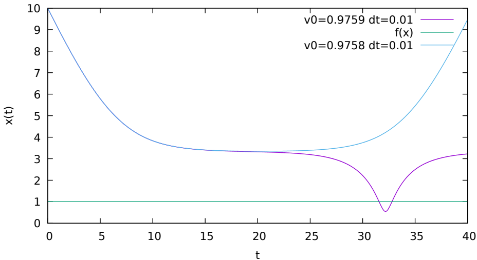
Velocita minima per raggiungere x=1 (algoritmo utilizzato leapfrog)
