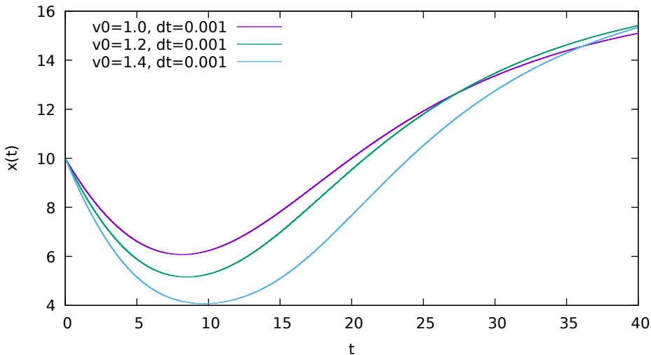
Componente d attrito, variazione traiettoria al variare di v_0 in [1.0, 1.4] (RK4)
