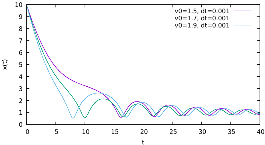
Componente d attrito, variazione traiettoria al variare di v_0 in [1.5, 1.9] (RK4)
