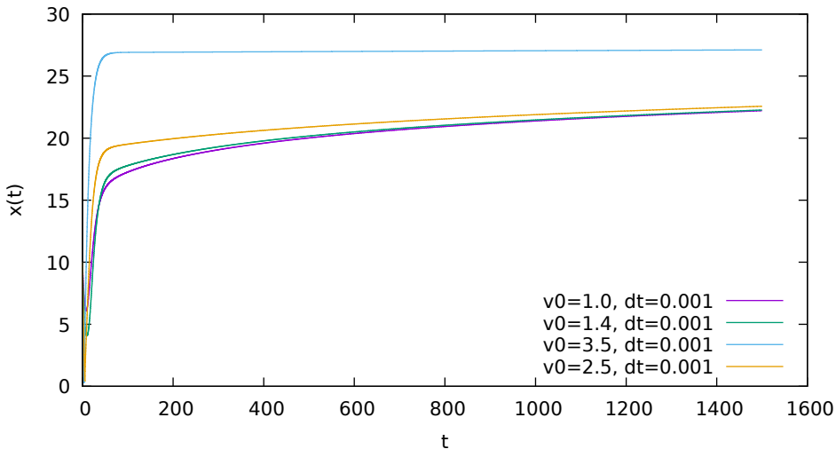
Componenete d attrito, traiettoria particella su tempi lunghi (RK4)
