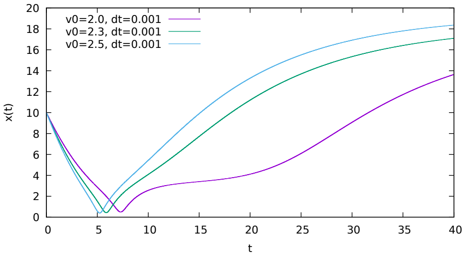
Componente d attrito, variazione traiettoria al variare di v_0 in [2.0, 2.5] (RK4)
