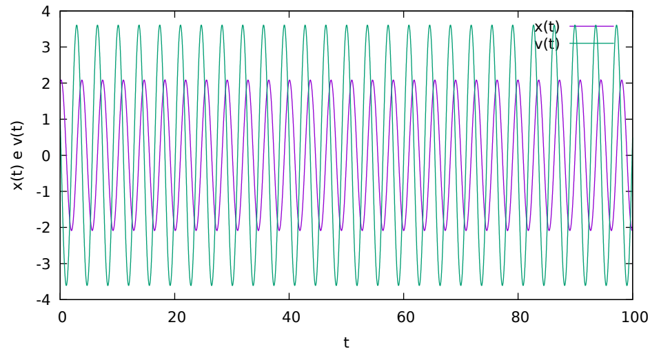
Runge-Kutta 4° ordine (dt=0.01)
