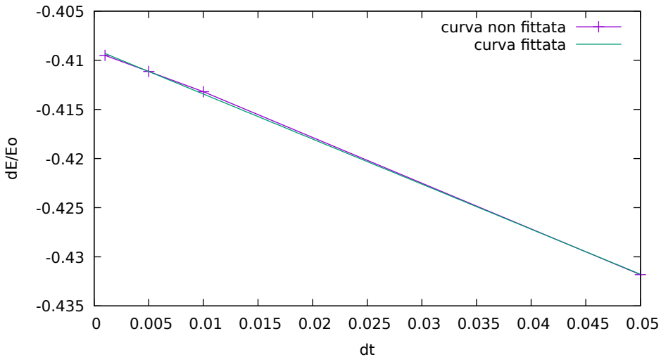
Andamento errore energia con Eulero-Cromer
