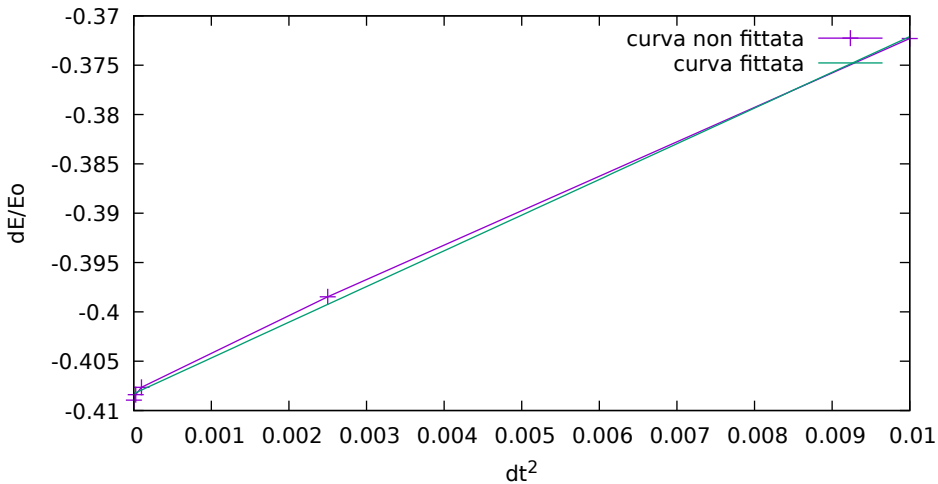
Andamento errore energia con Leap Frog
