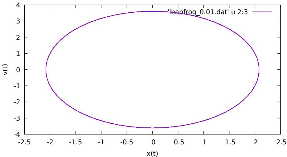
Leap Frog , Spazio delle fasi con dt=0.01
