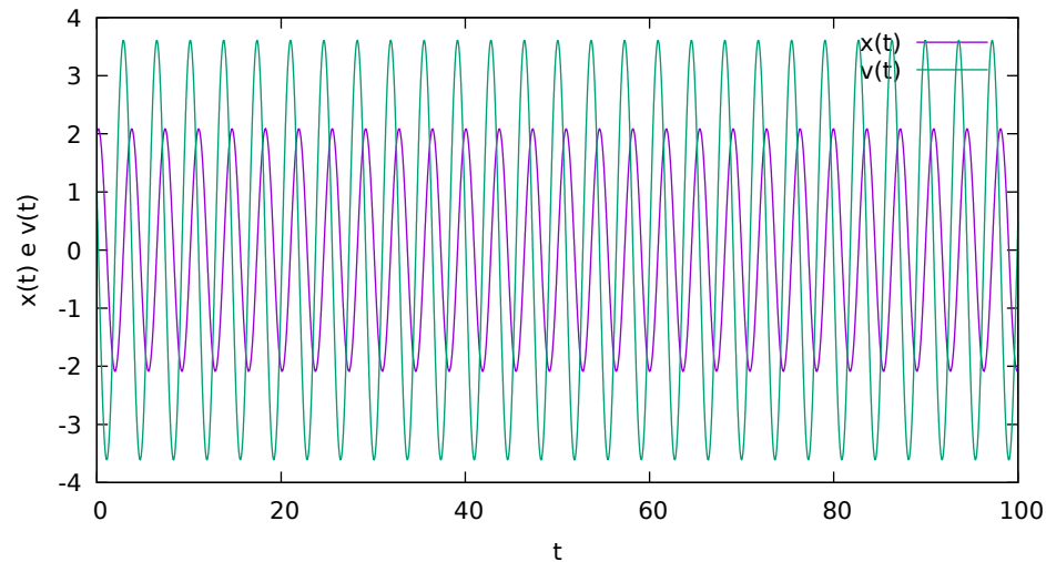
Verlet Velocita con dt=0.01
