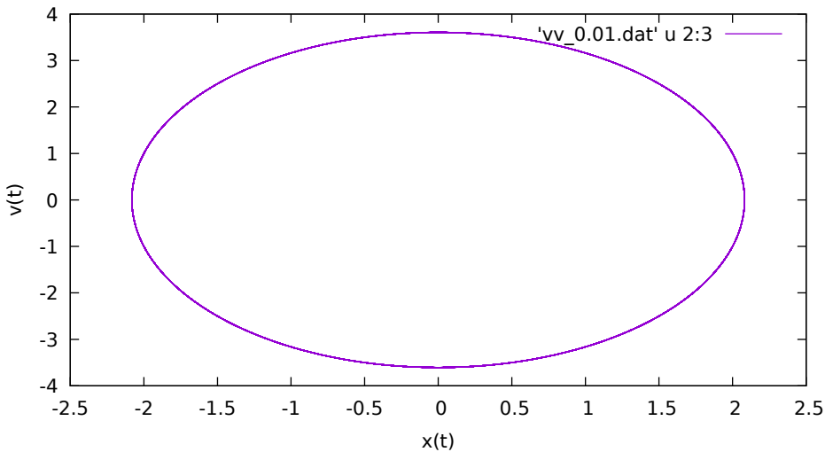
Verlet Velocita , Spazio delle fasi con dt=0.01
