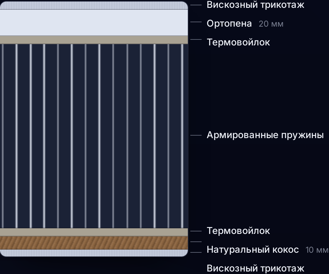
РАЗРЕЗ
