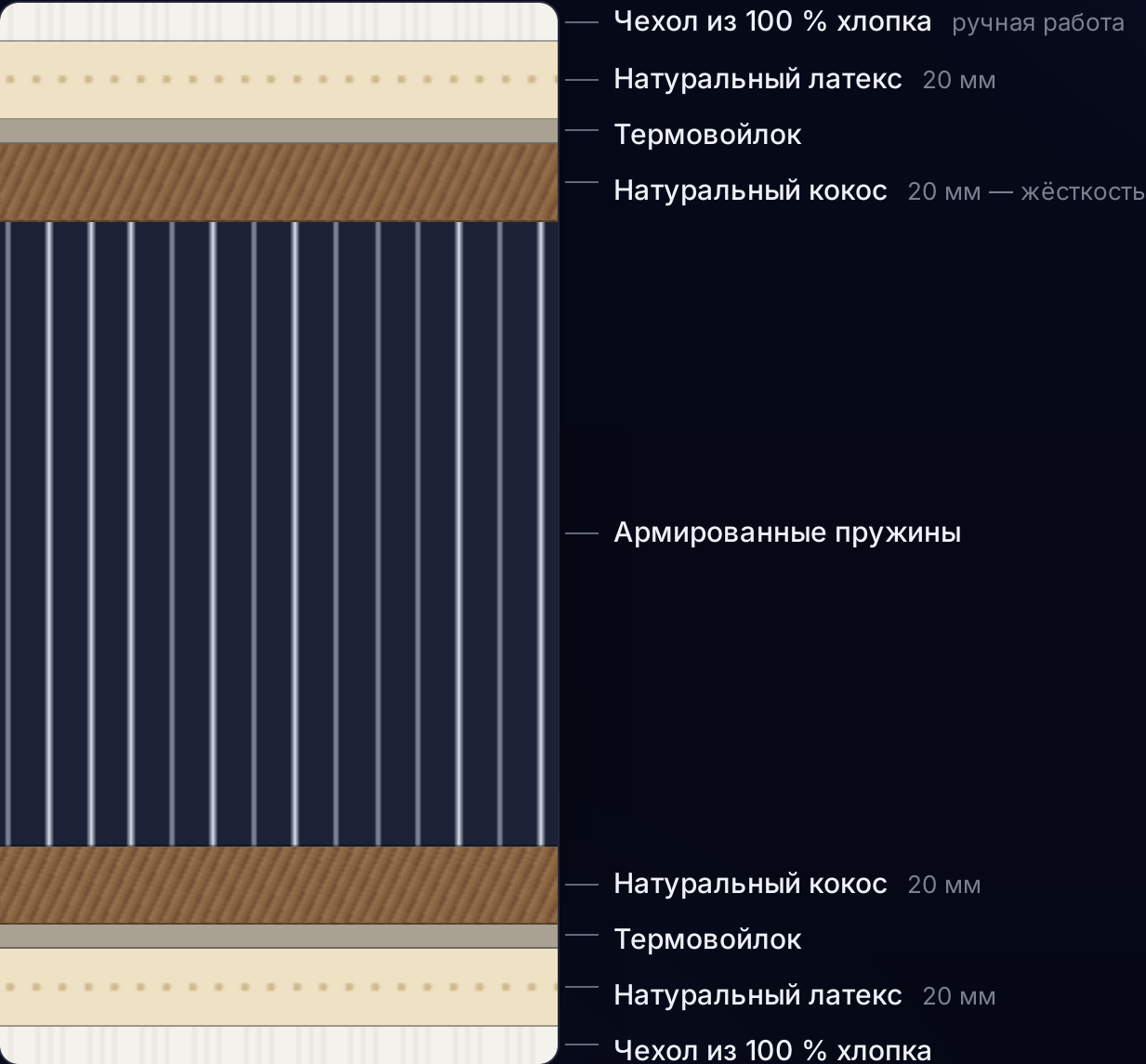
РАЗРЕЗ
