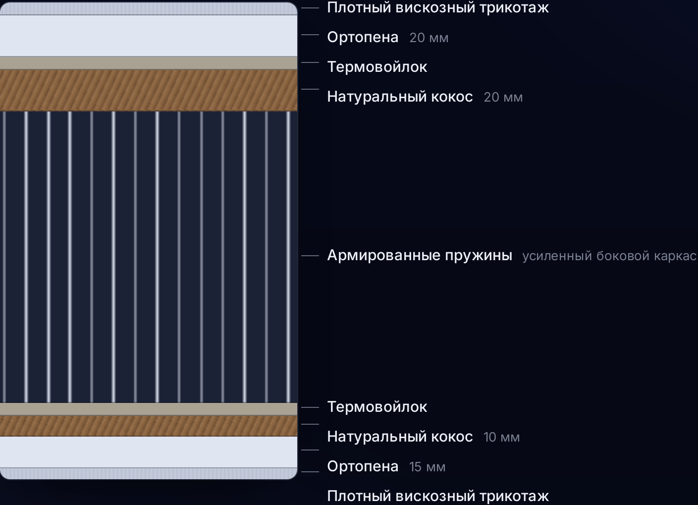
РАЗРЕЗ
