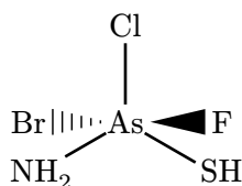
Trigonal bipyramidal · @TB5
