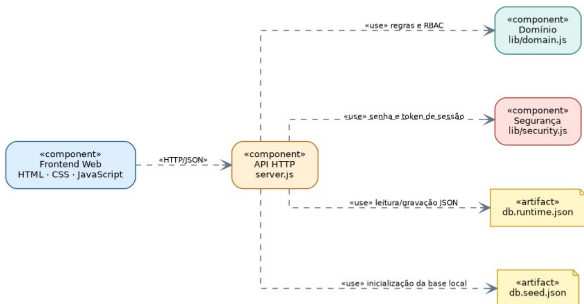
Figura 10 - Componentes efetivamente implementados no MVP.
