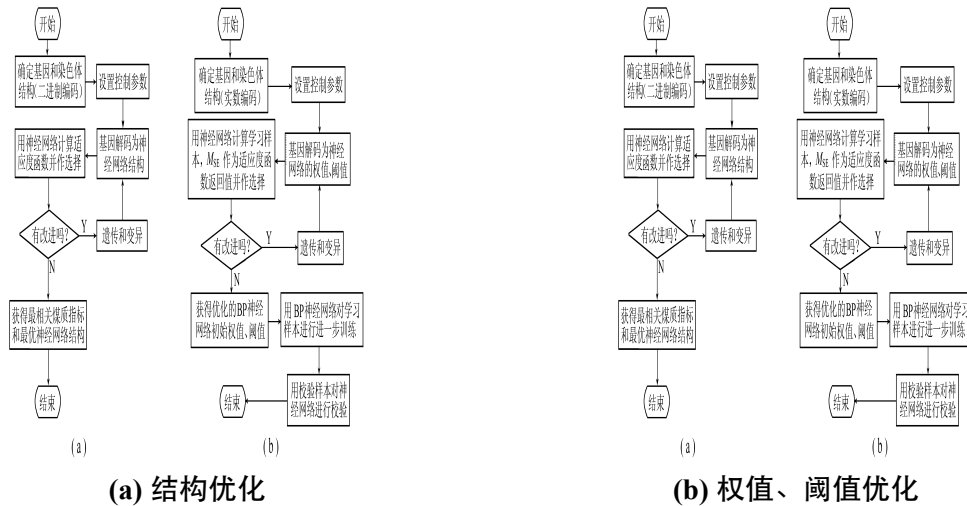
图 2.3 BP-GA 计算过程
