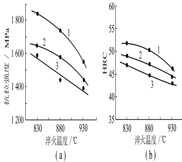
图 2.2 淬火温度对 25MnV 钢硬度的影响
