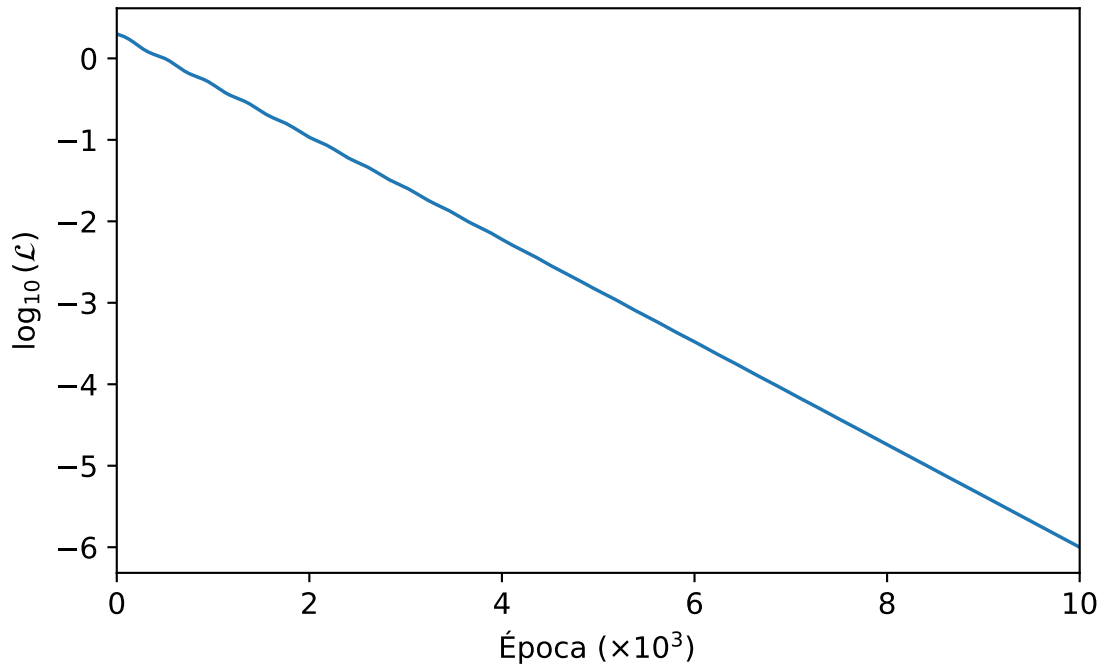
Curva de treinamento da PINN
