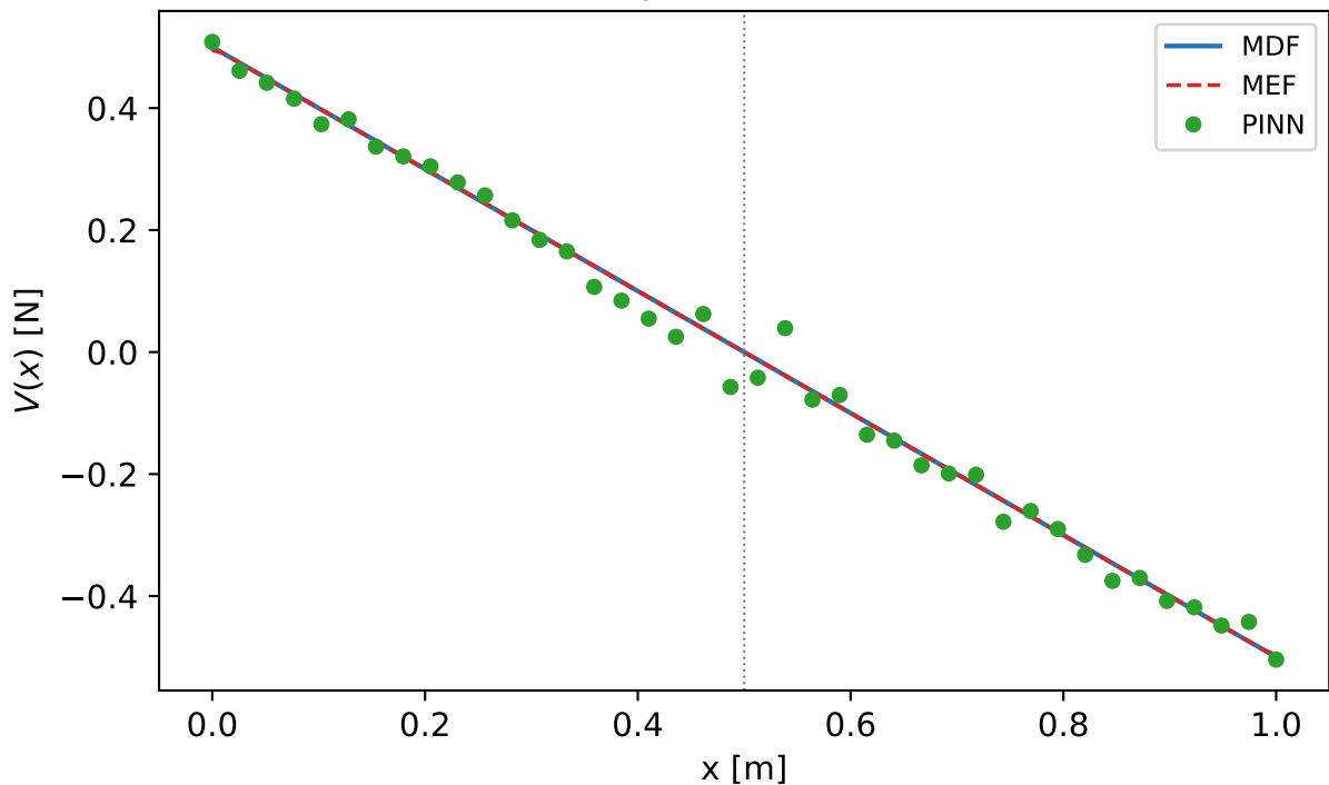
Esforço cortante V(x)
