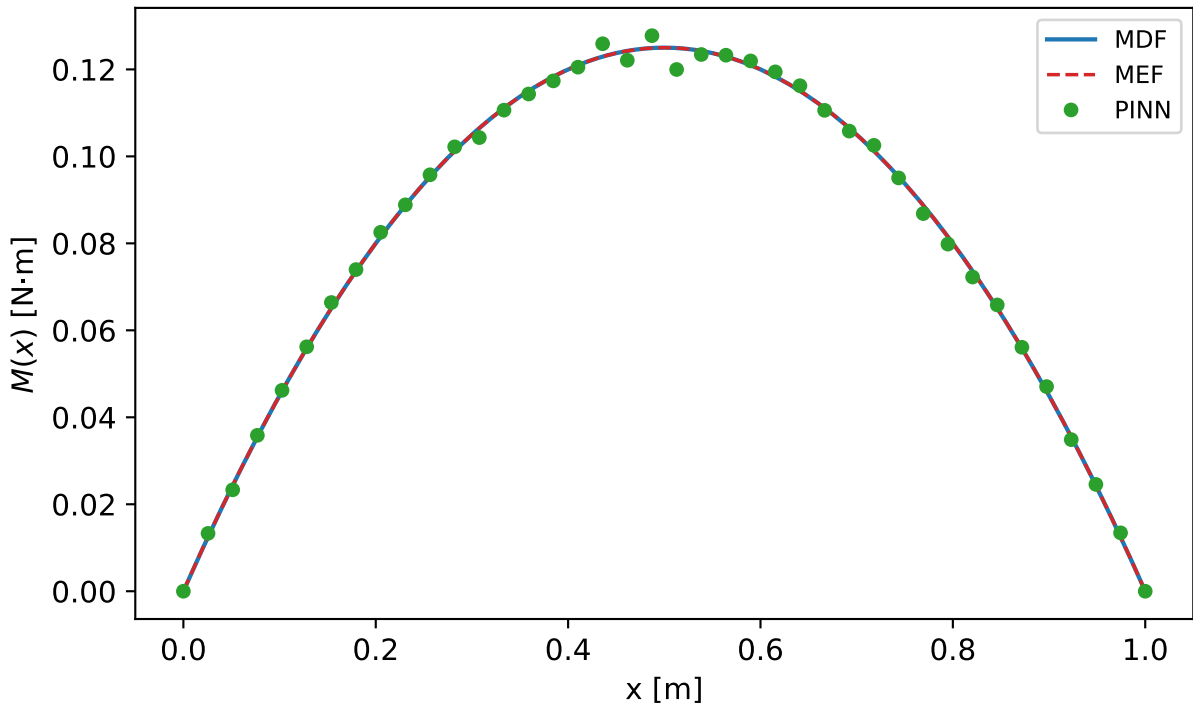
Momento fletor M(x)
