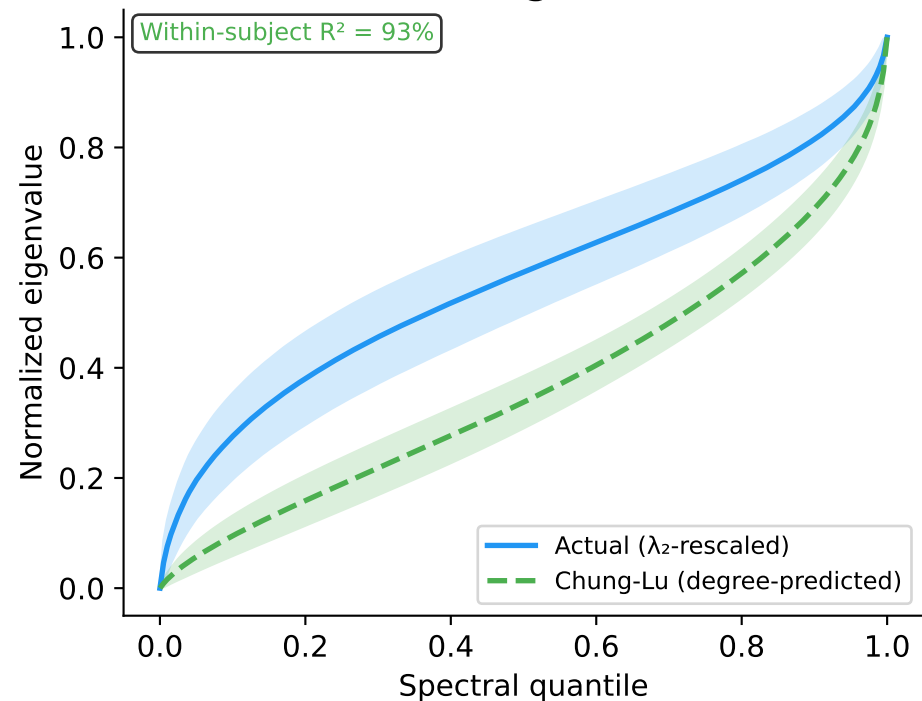
A. Actual vs Degree-Predicted
